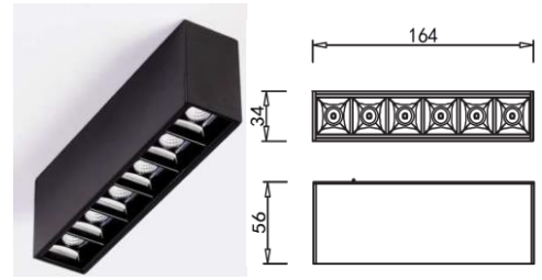
DOT06 12°/ 34°/ 48° Abstrahlwinkel DC 24V sand weiss/ sand schwarz Osram 8W >80Ra 2700k/ 3000k/ 4000k/ 5000k/ 6500k
