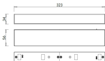
Linear32 323mm länge Diffuslicht DC 24V Osram 15W >80Ra 2700k/ 3000k/ 4000k/ 5000k/ 6500k sand weiss/ sand schwarz
