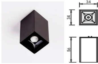
DOT01 12°/ 34°/ 48° Abstrahlwinkel DC 24V sand weiss/ sand schwarz Osram 1W >80Ra 2700k/ 3000k/ 4000k/ 5000k/ 6500k
