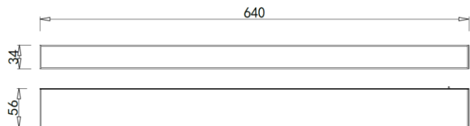
Linear64 640mm länge Diffuslicht DC 24V Osram 30W >80Ra 2700k/ 3000k/ 4000k/ 5000k/ 6500k sand weiss/ sand schwarz
