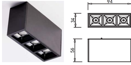
DOT03 12°/ 34°/ 48° Abstrahlwinkel DC 24V sand weiss/ sand schwarz Osram 4W >80Ra 2700k/ 3000k/ 4000k/ 5000k/ 6500k
